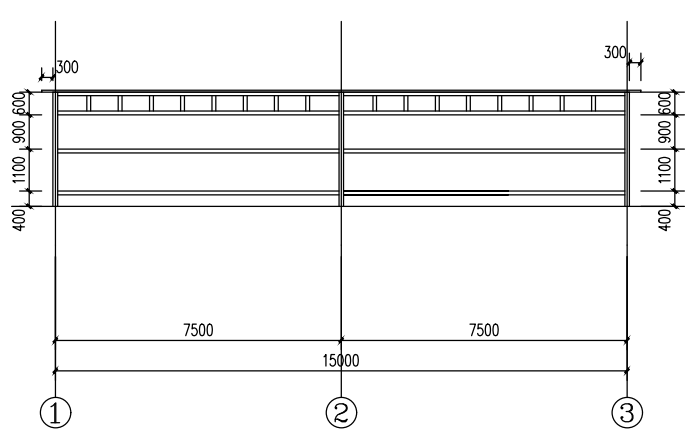
②轴立面图
