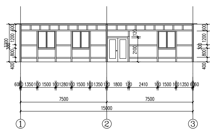
①轴立面图
